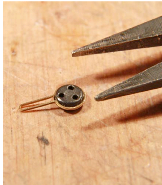
An den Juffern die Plastikbügel entfernt und die Eisen mit Hilfe der Flanken einer feinen Zange darüber gedrückt und darauf achten, dass das mittlere Loch nach unten zeigt ...
