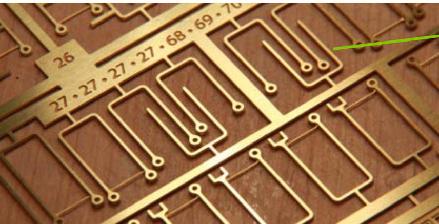
Abstützung des vordersten Poopdeckhalters ankleben. (Hinweis: Die Stütze ist etwas länger als auf diesem Bild!)
